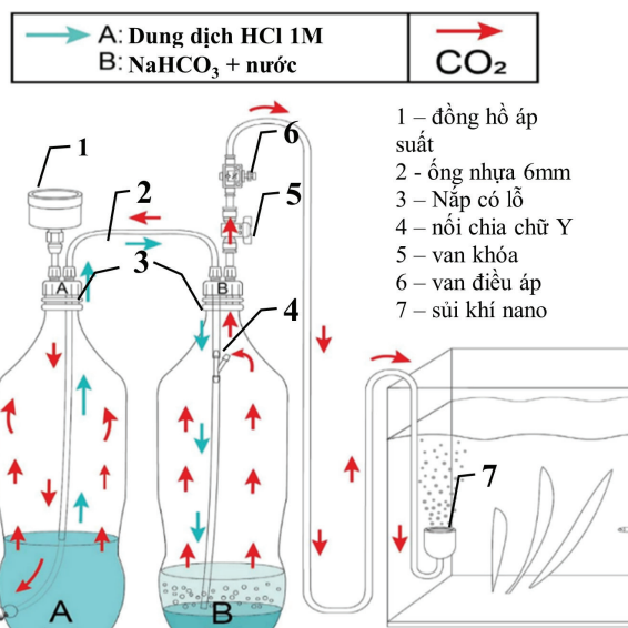
Bộ kit “Hệ thống tạo khí CO 2 ” và Sơ đồ thiết kế và vận hành.
